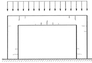
1. 鉛直荷重による柱及び梁の曲げひび割れ
