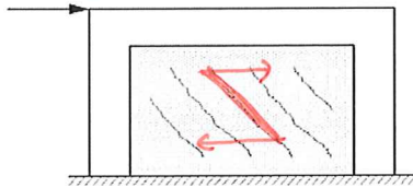
3. 水平荷重による耐力壁のせん断ひび割れ
